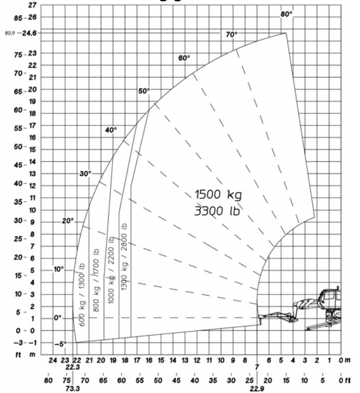
Rotatie op verlaagde stabilisatoren met 1500 kg giek
